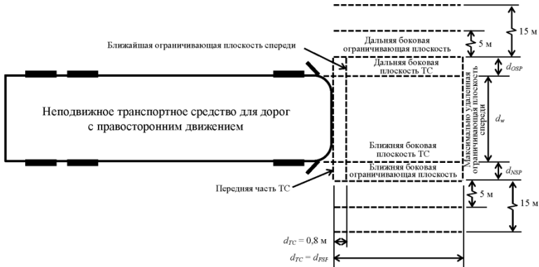
Рис. 1 Схема статических испытаний с пересечением
