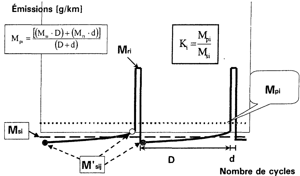
Figure 8/1 : Paramètres mesurés lors des essais d'émissions pendant et entre les cycles où se produit une régénération (il s'agit d'un exemple : les émissions pendant la période "D" peuvent en fait augmenter ou diminuer)
