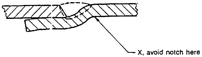
joggle weld
